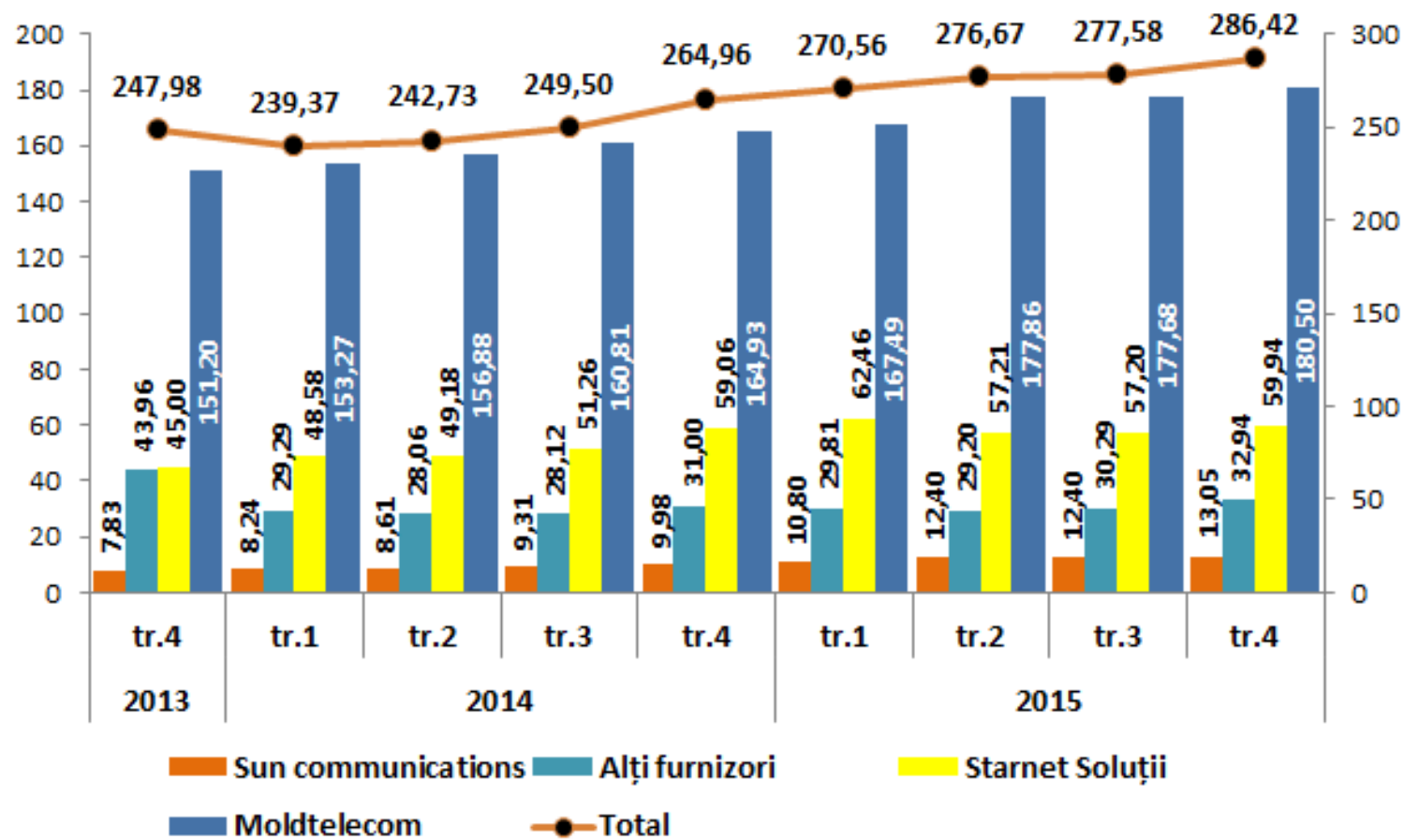
Fig. nr. 1. Structura pieței în funcție de veniturile obținute de furnizori
